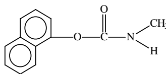
Carbaryl
