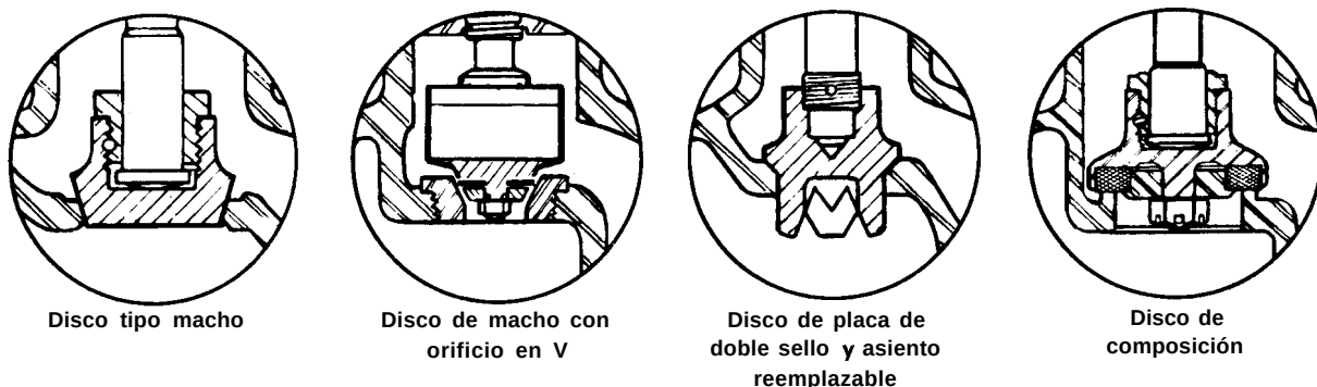
Fig. 12 Discos de diversos tipos para válvulas de globo
