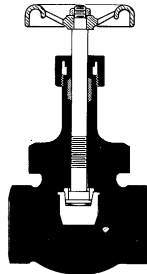
Fig. 8 Válvula de globo con macho, con vástago elevable
