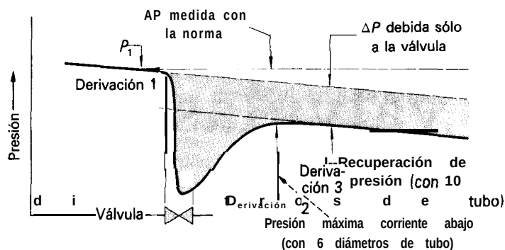
Fig. 5 La caída de presión alrededor de una válvula abierta se debe a las pérdidas en el tubo y en la válvula
