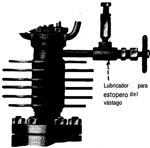
Bonete con aletas (Para temperaturas mayores de 400°F)
