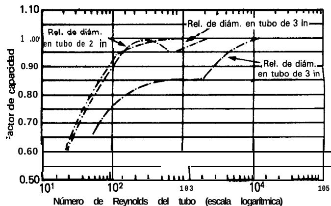
Fig. 4 El flujo en el conducto de un medidor de mira puede tener comportamiento anómalo en la región de transición
