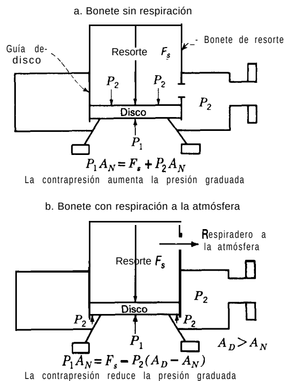
Fig. 2 Fuerzas sobre el disco de válvula de desahogo convencional
