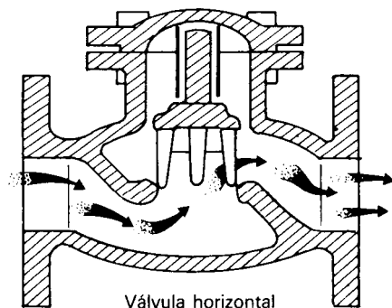
Fig. 6 Las válvulas de retención impiden la inversión del flujo
