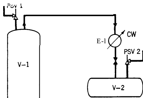
Fig. 9 Las unidades bloqueadas requieren válvulas de desahogo separadas
