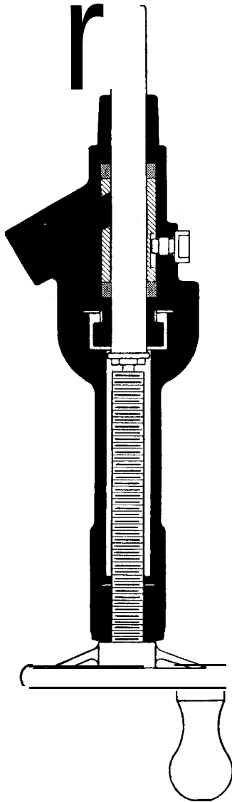
Fíg. 7 Válvula manual para muestreo
