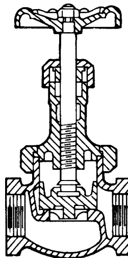
Fig. 1 Válvula de globo con asiento metálico
