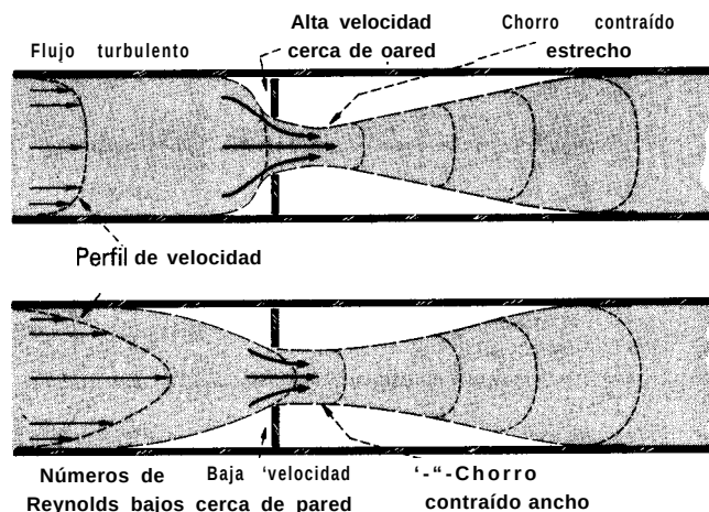
Fig. 1 Con flujo turbulento, los chorros contraídos son más estrechos que los obtenidos con números de Reynolds más bajos
