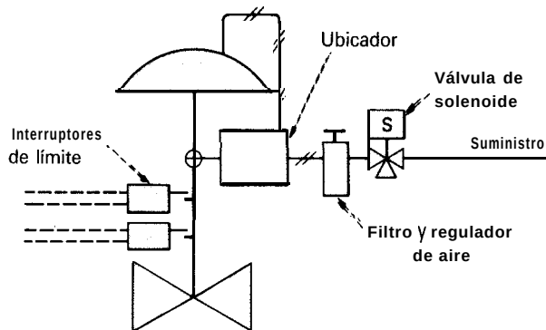
Fig. 3 Los ciclos de trabajo gastan los componentes auxiliares
