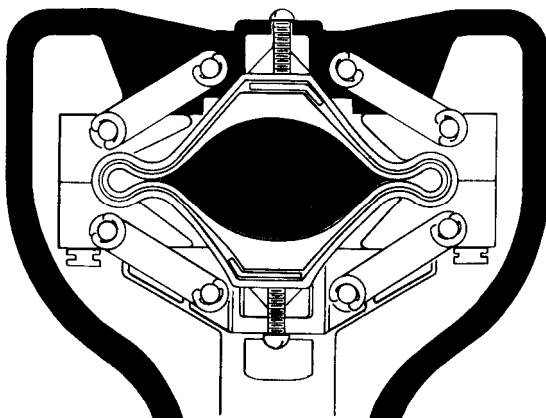
Fig. 14 Una válvula flexible que incluye un tubo preformado
