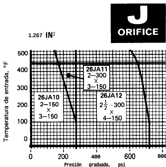
Fig. 6 Sección de una gráfica típica para selección en el catálogo de un fabricante
