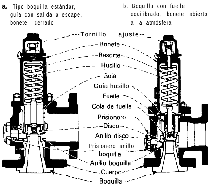
Fig. 1 Nomenclatura de válvulas de desahogo de seguridad típicas
