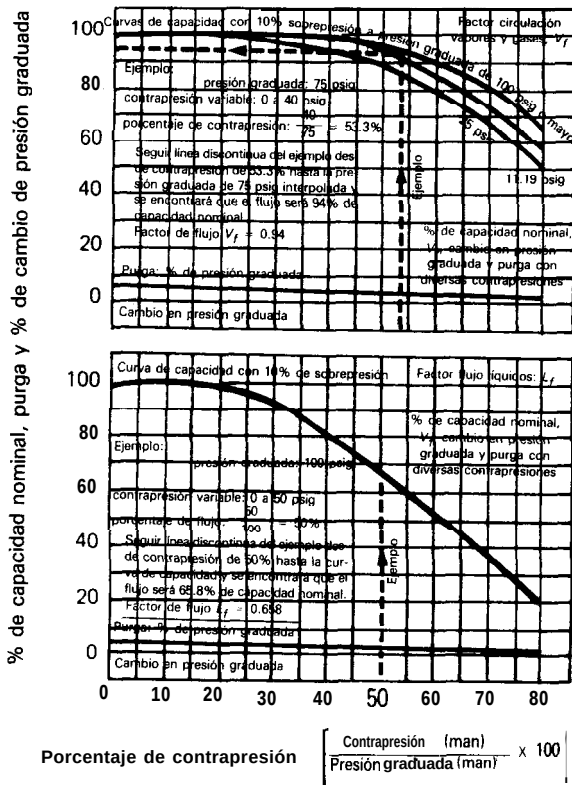
Fig. 10 Características de rendimiento de válvulas de fuente de presión equilibrada
