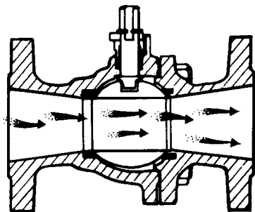
Fig. 3 La válvula de bola abierta permite flujo sin restricción
