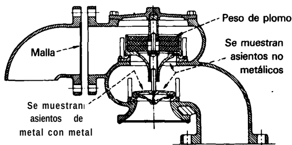
Fig. 8 - Respiradero para tanques de almacenamiento atmosférico
