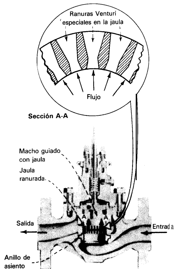
Fig. 9 Las trayectorias múltiples generan menos ruido
