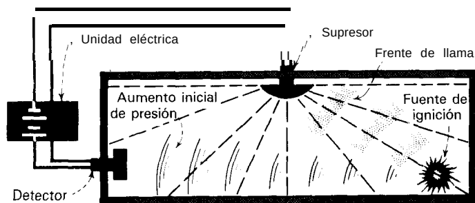
Fig. 14 El detector capta el aumento inicial de presión
