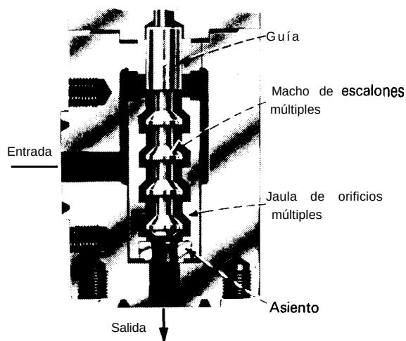
Fig. 4 La válvula con guarnición escalonada distribuye la caída de presión
