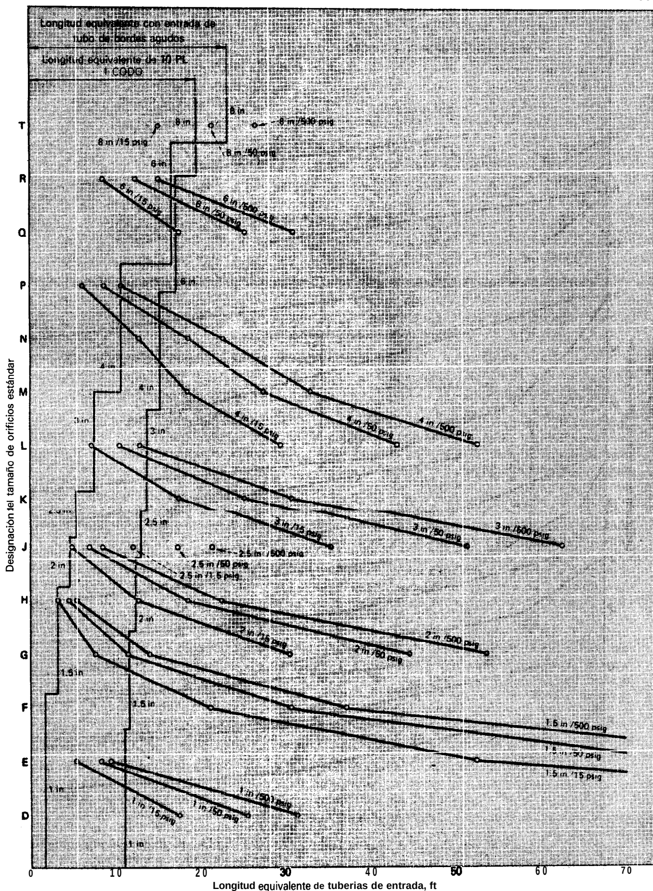
Fig. 2 Longitud equivalente de tubería de entrada permitida por los códigos para válvulas de desahogo convencionales, de fuente equilibrado y operados con piloto con derivación local
