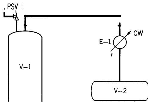
Fig. 8 Componentes interconectados tratados como una unidad
