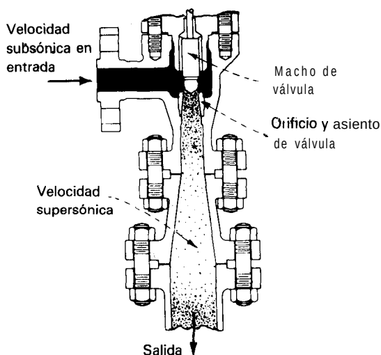
Fig. 1 La válvula en ángulo convencional tiene flujo supersónico
