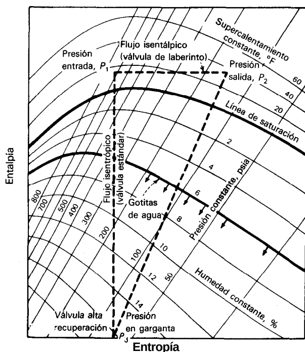
Fig. 2 La estrangulación isentrópica crea gotitas de agua
