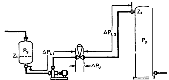
Fig. 3 Sistema típico de flujo de líquidos
