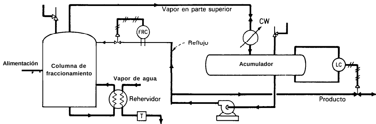
Fig. 12 La columna de fraccionamiento puede tener sobrepresión por bloqueo, pérdida de agua, falta de equipo o instrumentos
