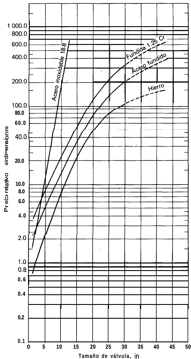
Fig. 23 Costos no instalados, relativos, de válvulas de compuerta para 150 psi, extremos con brida, discos de cuña, vástagos elevables
