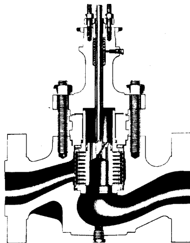
Fig. 6 Válvula con guarnición para AP de 1 000 a 3 000 psi
