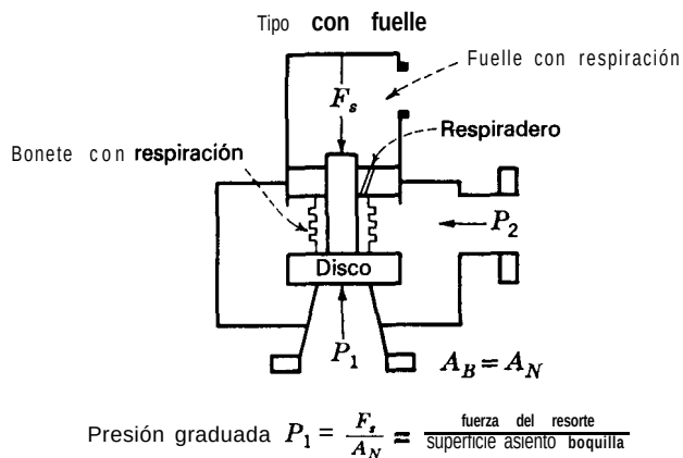
Fig. 3 Fuerzas en el disco de válvula de fuelle equilibrado
