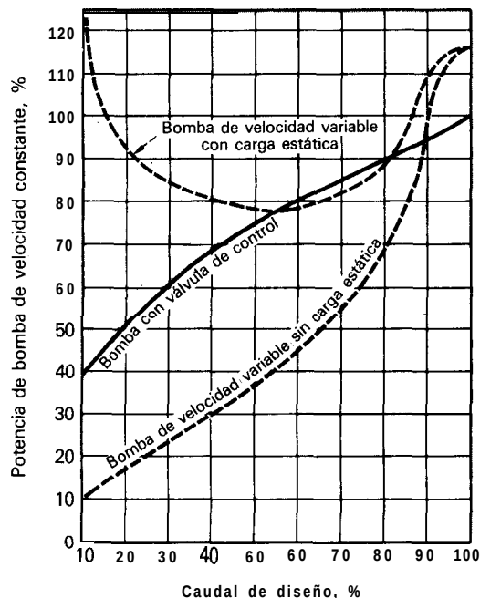
Fig. 4 Potencia para bomba de velocidad variable comparada con la de una de velocidad constante con válvula
