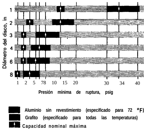
Fig. 3 Exactitud del disco con mínima presión de ruptura
