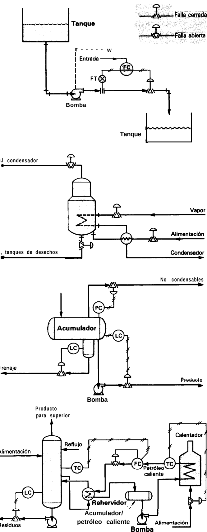
Fig. 5 La posición de falla sin peligro de las válvulas de control se debe indicar con claridad en los diagramas
