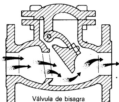
Válvula de bisagra
