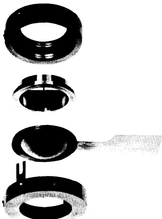
Fig. 7 El disco de ruptura descarga las explosiones
