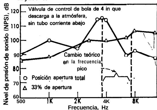
Fig. 5 Frecuencias pico de válvulas de control en relación con la vibración de la tubería adyacente
