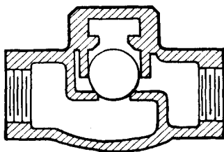
Fig. II Las válvulas de retención de bola no suelen tener problemas de servicio
