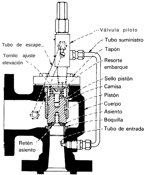
Fig. 4 Válvula de desahogo de seguridad operada por piloto
