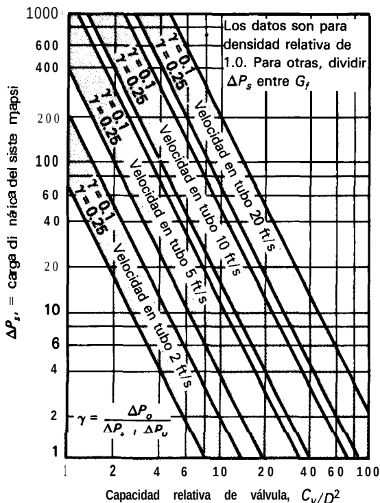
Fig. 1 Determinación de capacidad relativa de válvula de control
