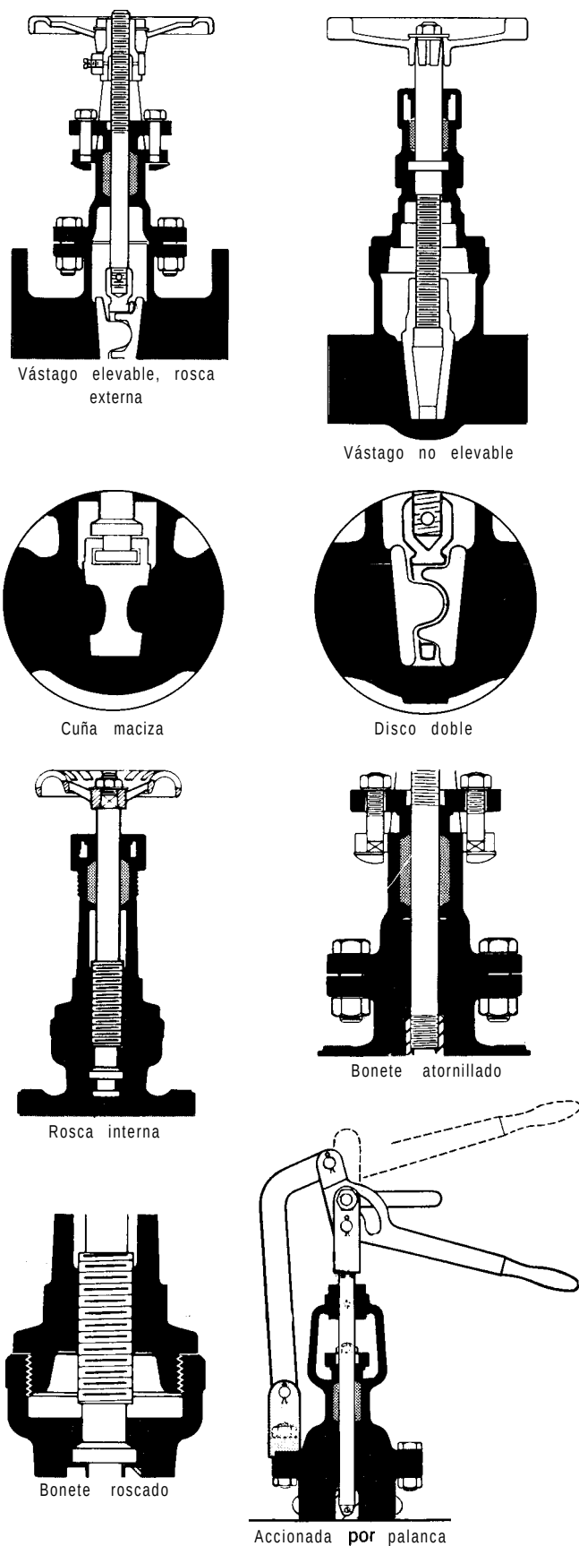
Fig. 3 Algunas de las muchas variantes de tornillos, bonetes y discos de válvulas de compuerta
