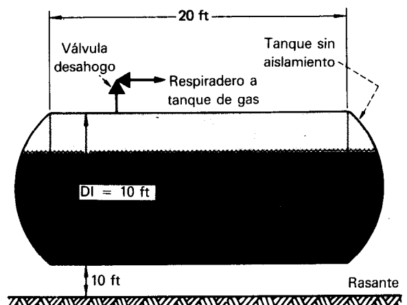
Fig. 2 Diseña y dimensiones del tanque de almacenamiento
