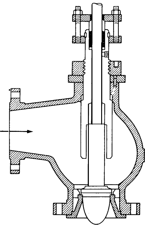
Fig. 4 Válvula de reducción para servicio moderado, el cuerpo ampliado reduce la velocidad; si se coloca un orificio en la salida se reducen los daños en el cuerpo por la corriente de descarga; el asiento especial de dos piezas se dilata en sentido radial ( ITT Conoflow )
