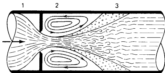
Fig. 2 El líquido a alta velocidad que pasa por la restricción induce una sección de baja presión en el chorro contraído. Hay presiones todavía más bajas en los vórtices creados en la capa límite del chorro
