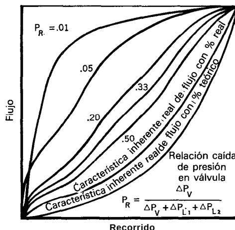
Fig. 6 Características real e inherente de flujo
