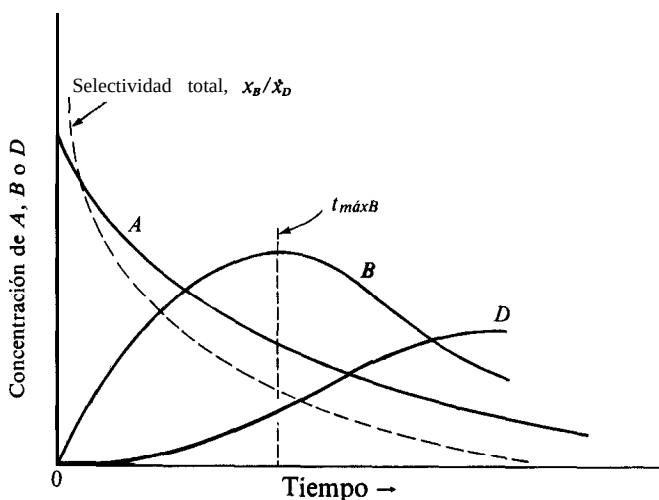
Fig. 2-7 Concentraciones en función del tiempo para el sistema de reacciones consecutivas A \rightarrow B \rightarrow D para B = D = \text{Oat} = 0 .
