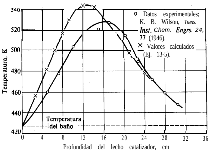
Fig. 13-10. Perfil longitudinal de temperaturas de un reactor para la hidrogenación de nitrobenzeno.
