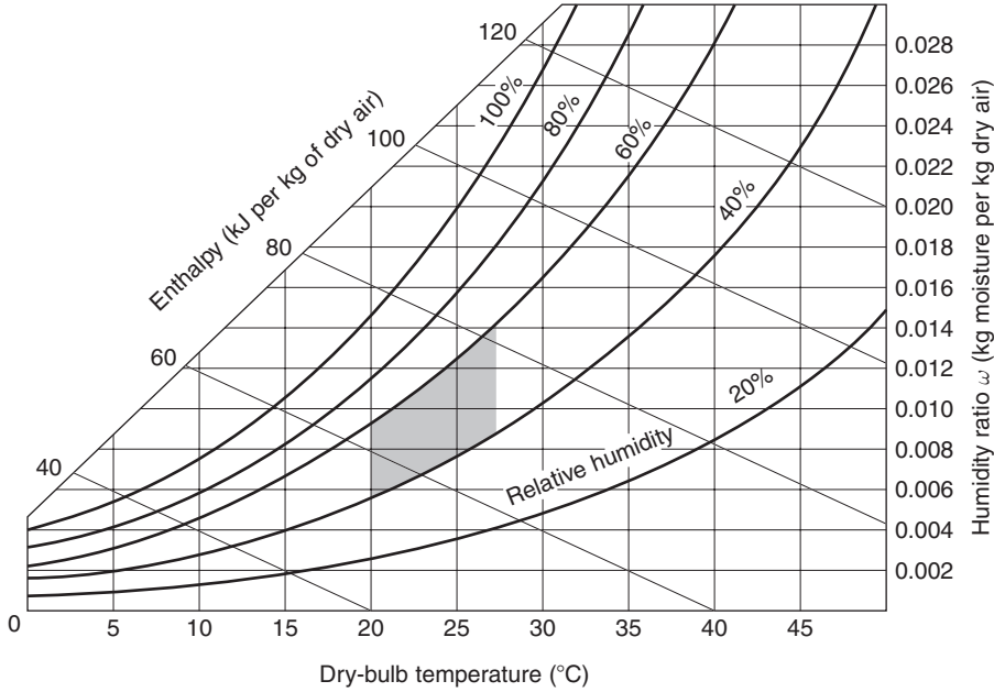
Fig. 6.4. Psychrometric chart.
