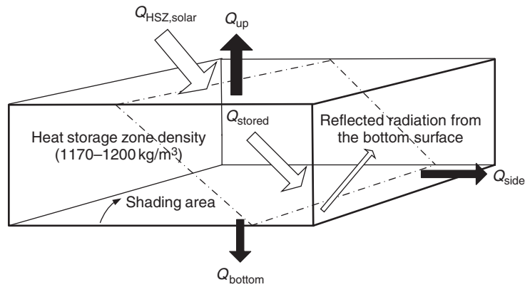
Fig. 10.11. HSZ of the solar pond.
