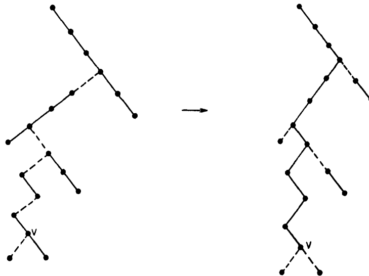
FIG. 5.3. Exposing a vertex v .
