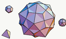
Figura 3.4. Poliedros
