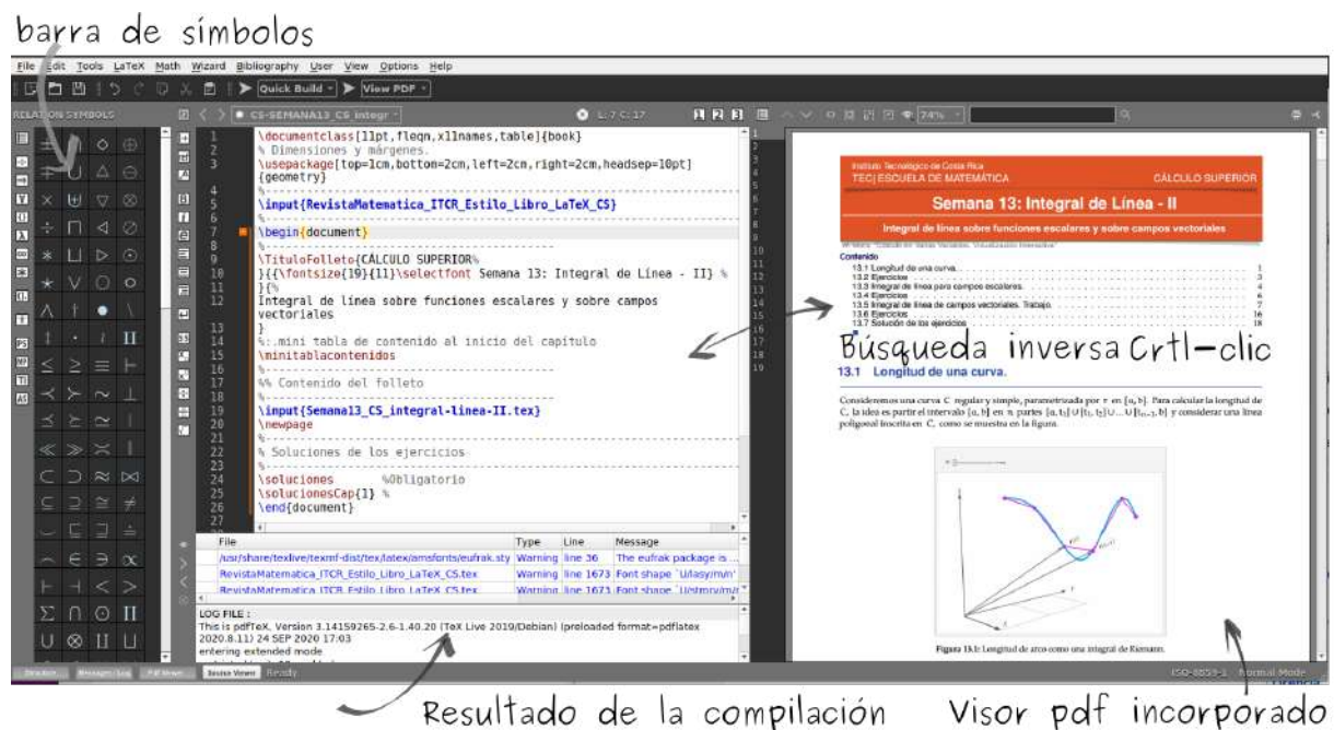
Figura 1.3. Editor TexMaker
