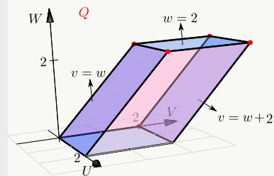
Figura 6.1. Un paralelepípedo
