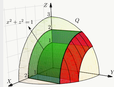
Figura 6.2. Sólido Q
