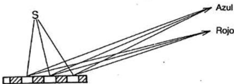
Figura 27. Una red de difracción con surcos a la distancia adecuada para la luz roja, también funciona para otros colores si el detector se coloca en un lugar diferente.
